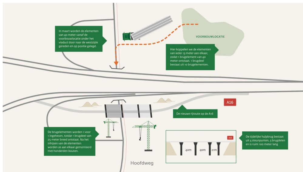
Afbeelding: bouwproces tijdelijke hulpbrug
